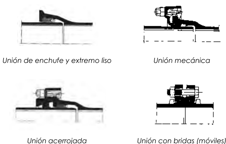
Figura AI-13. Tipos de uniones en tubos de función
