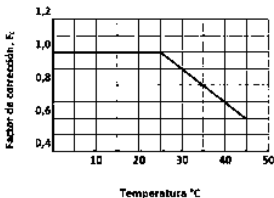
Figura AI-26. Tubos de PVC-U. Factor de corrección de PN por la Tª (UNE-EN 1.456-1)
