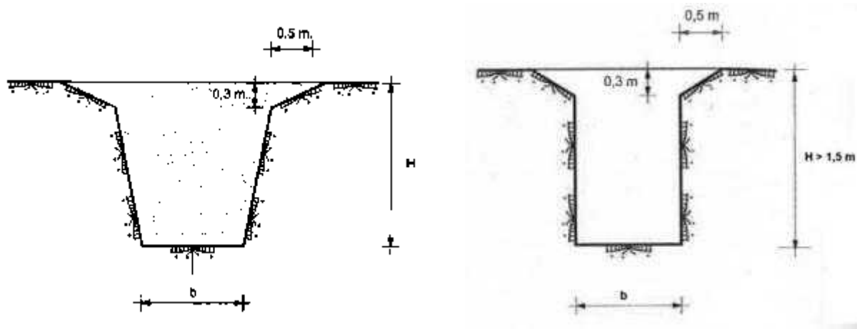
Bordes ataluzados en zanjas sin entibar
