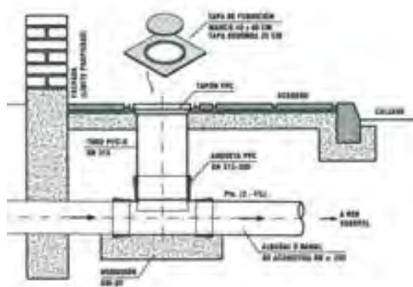
Figura III-4. Arqueta de arranque con registro PVC de paso directo
