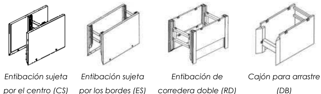
Figura V-4. Sistemas de entibación no estructural
