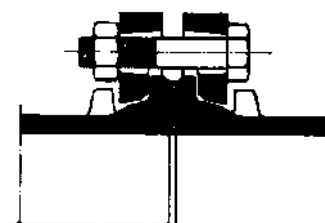
Unión con bridas (móviles)
