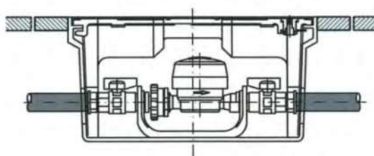
TRAMPILLÓN CON CONTADOR
