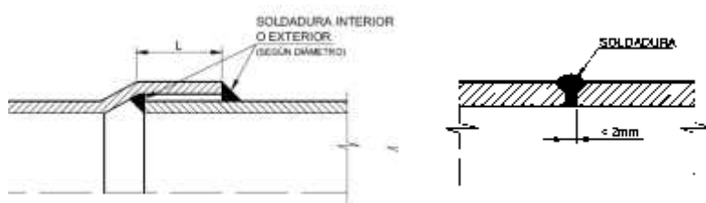
Unión abocardada
