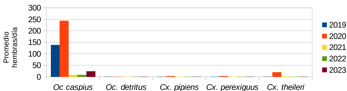
Fig. 1. Dinámica de poblaciones de las principales especies plaga registrada en la estación de muestreo de Matalascañas: N.º medio de hembras mosquitos/jornada en trampa CDC+CO 2 .
